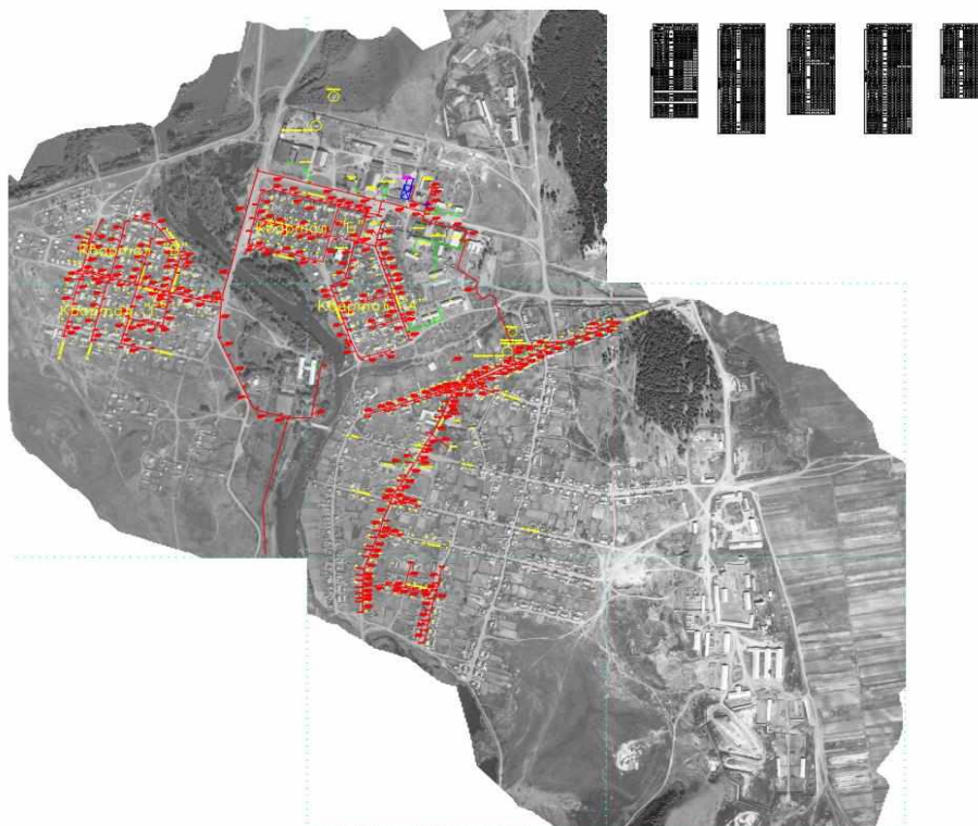
Схема теплоснабжения с. Тесь
