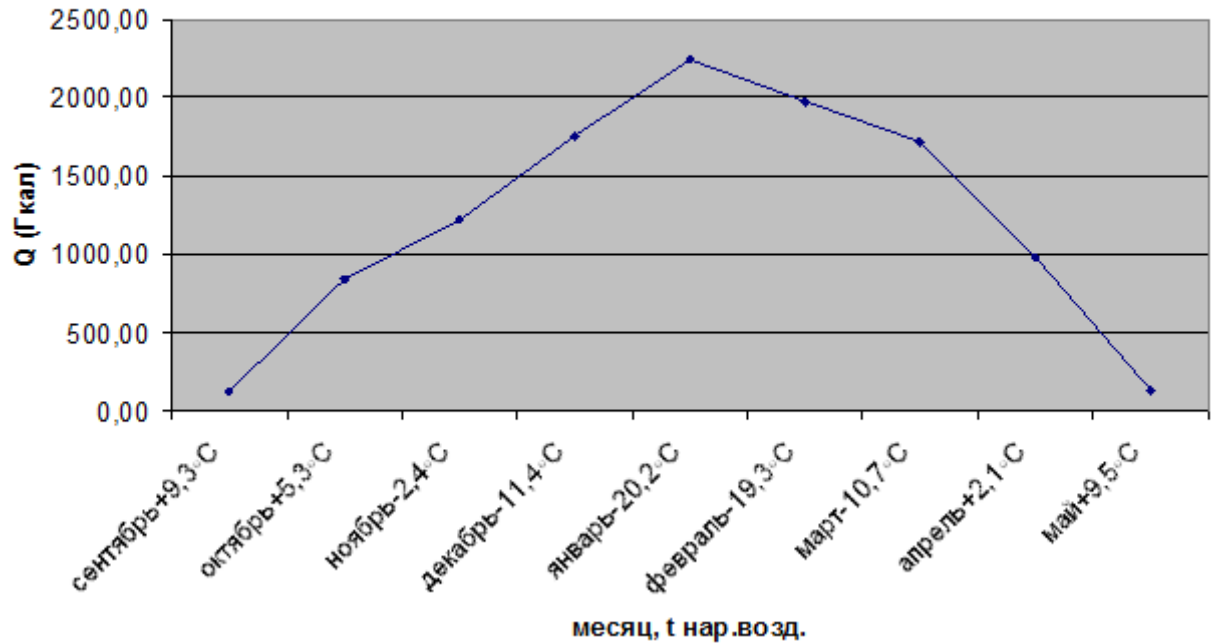
График годовых тепловых нагрузок по котельной с. Лугавское
