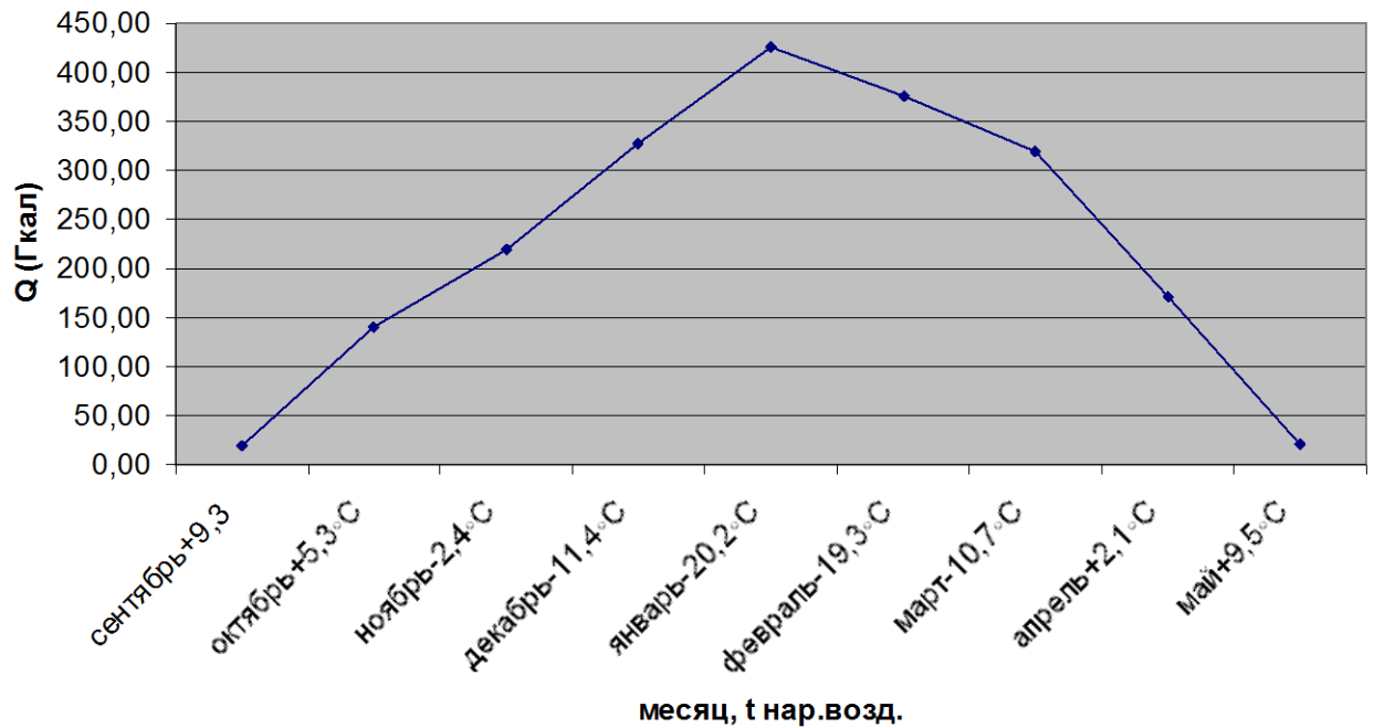
График годовых тепловых нагрузок по котельной с. Знаменка школа
