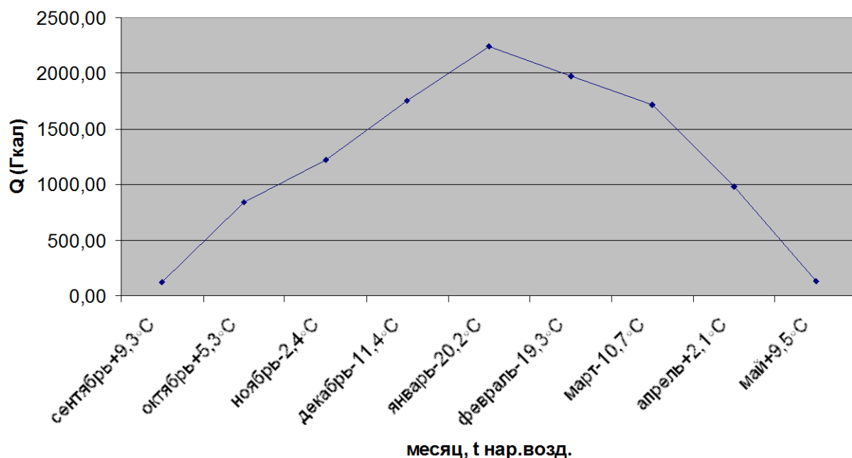
График годовых тепловых нагрузок по котельной с. Лугавское
